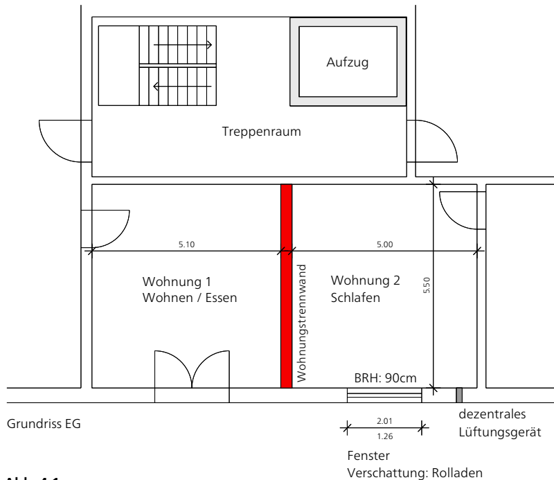
Abb. 4.1: Grundrissituation der Beispielbemessung
